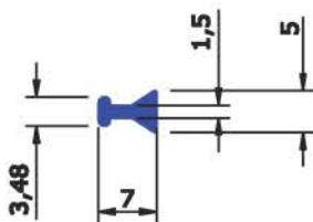
SEC No : 4062 WEIGHT Kg/Mtr 0.180 - 0.230
