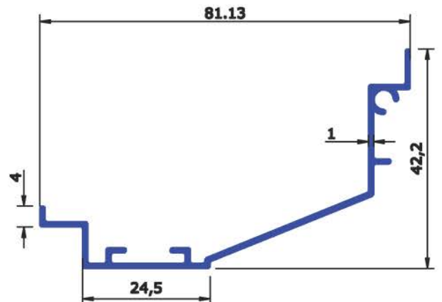
SEC No : 4065 WEIGHT Kg/Mtr 1.400 - 1.500
