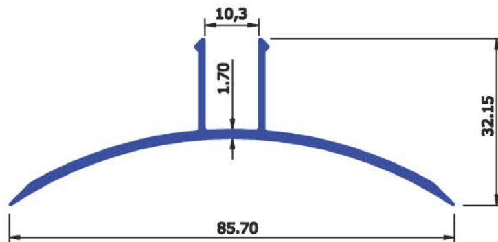
SECTION No : 5209 WEIGHT Kg/Mtr : 0.516
