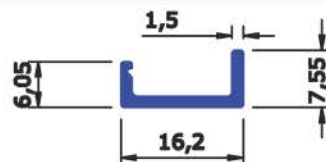
SEC No : 6563 WEIGHT Kg/Mtr 0.106
