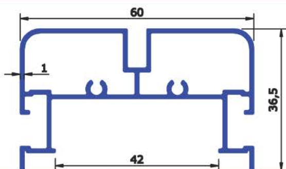
SEC No: 6752 WEIGHT KG/Mtr 0.700
