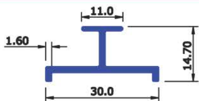
SEC No : 6404 WEIGHT Kg/Mtr 0.226
