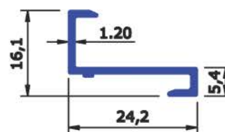
SEC No : 6410 WEIGHT Kg/Mtr 0.155
