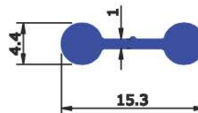
SEC No : 6323 WT RANGE Kg/12' : 0.095
