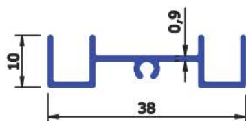
SEC No : 6147 WEIGHT Kg/Mtr 0.199
