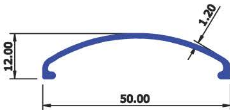
SEC No : 6123 WEIGHT Kg/Mtr 0.214
